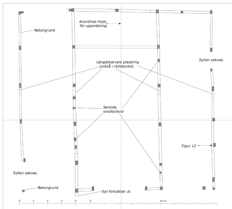
FIGUR 8. Planritningen visar att byggnaden idag har en nästan kvadratisk plan. Syllen är på flera ställen bort-ruttnad och på västsidan är den delvis ersatt av gjuten betong. Utmed norra gaveln finns en syll i ek, som ursprungligen kan ha varit genomgående, men som idag är avkapad i porten. Uppmätning och renritning Ulrik Hjort Lassen.
